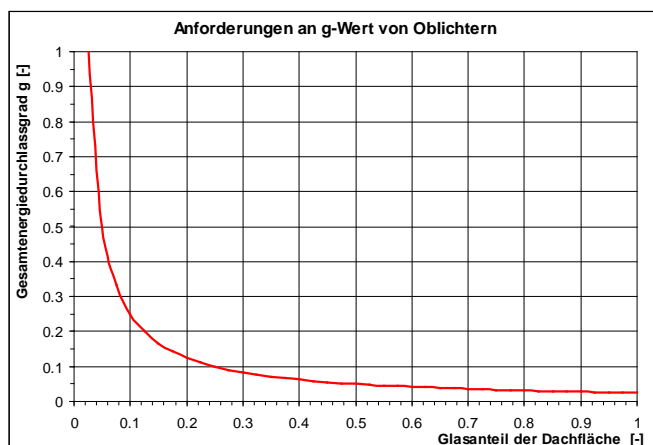
Abbildung 8: Anforderungen an den Gesamtenergiedurchlassgrad g von Oberlichtern
