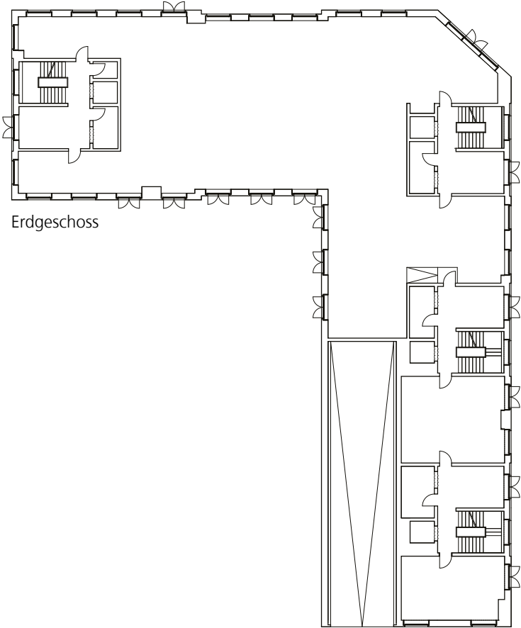
Mehrfamilienhaus an der Lenzburgerstrasse 1:400
