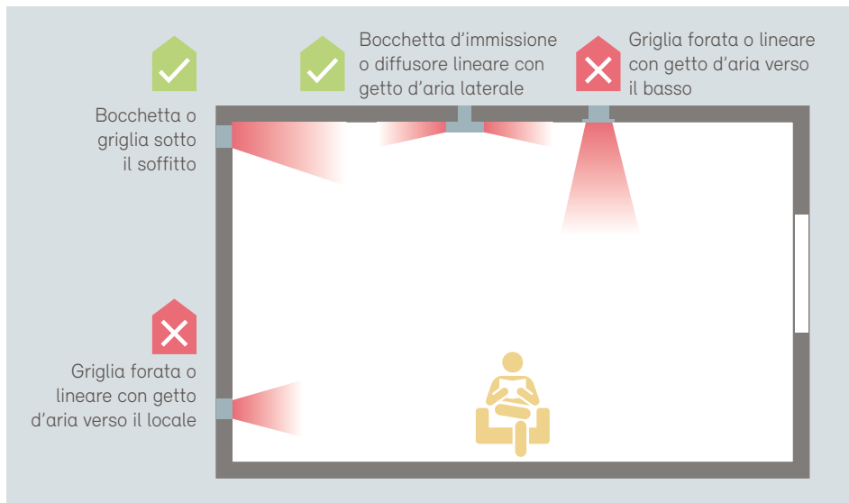
Disposizione corretta e non dei dispositivi d'immissione dell'aria.
