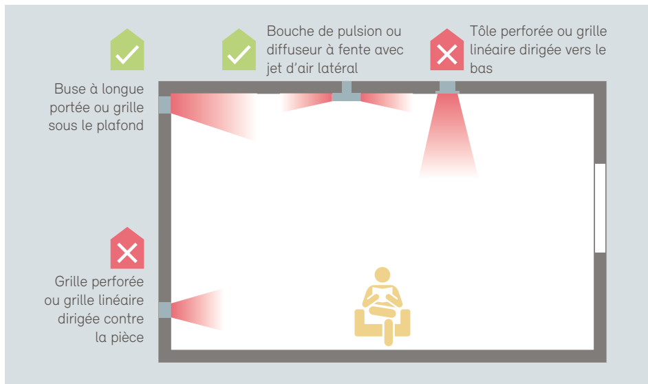
Disposition appropriée et non appropriée pour les bouches de pulsion.
