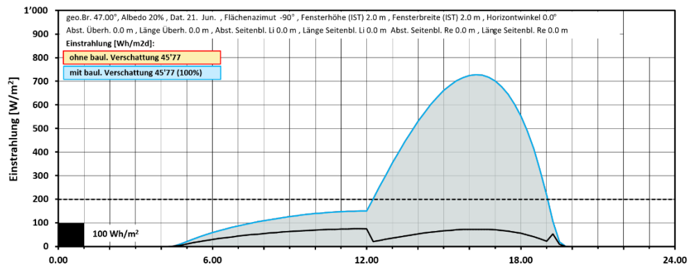
Figure 20 : diagramme d'irradiation ouest le 21 juin
