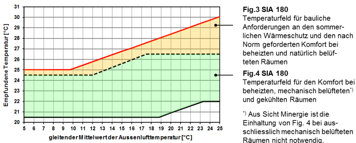
Figure 6: Comparaison des exigences selon la norme SIA 180
