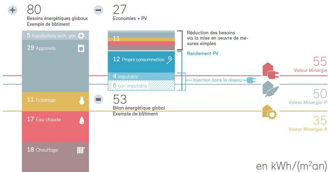
Figure 3 : Bilan et indice Minergie sur l'exemple d'un immeuble collectif, avec les exigences concernant l'indice Minergie pour le standard de base Minergie et le standard Minergie-P. Les valeurs des besoins standards additionnées sont présentées en parallèle des économies réalisées à la suite de mesures d'efficacité énergétique mises en place dans chaque secteur et du rendement de l'installation photovoltaïque obligatoire lors des nouvelles constructions. Toutes les valeurs sont exprimées en énergie finale, pondérée avec les facteurs de pondération Minergie.
