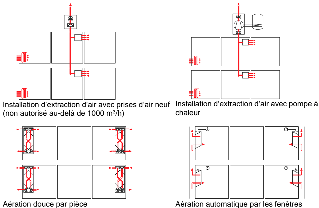
Figure 32 : Choix des installations de ventilation comme « type d'installation de ventilation standard »
