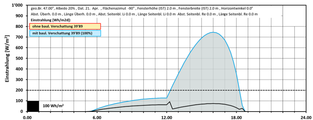
Figure 23 : diagramme d'irradiation ouest le 21 avril
