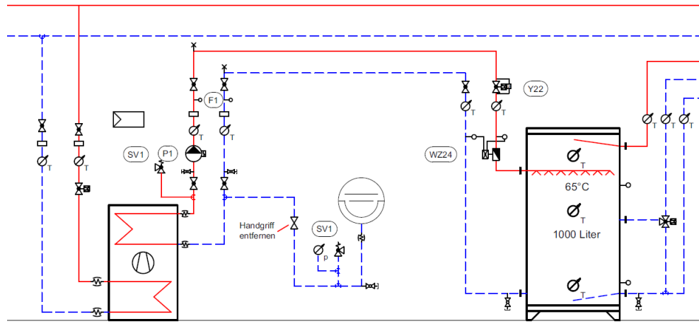
Figure 38 : Schéma booster ECS
