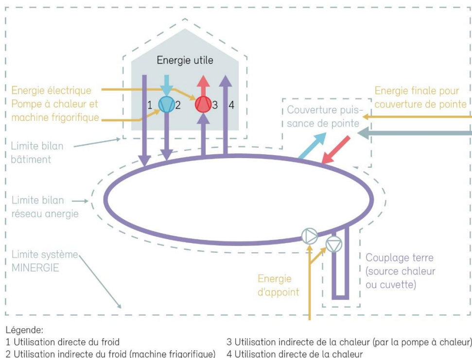
Figure 29 : Principe de calcul de l'énergie dans le standard Minergie
