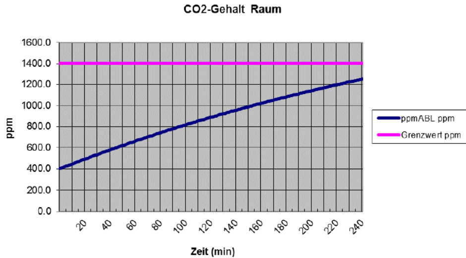
Figure 36 : Teneur en CO 2 pour deux personnes
