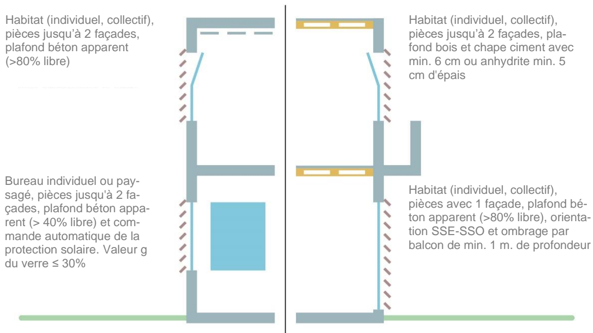
Figure 8: Cas standard pour les bâtiments résidentiels (Variante 1)
