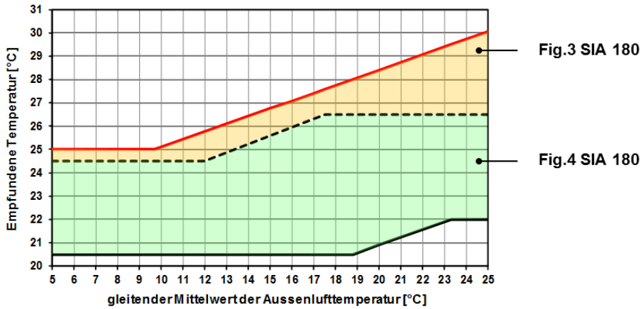
Figure 17: Fig. 3 et Fig.4 de la norme SIA 180
