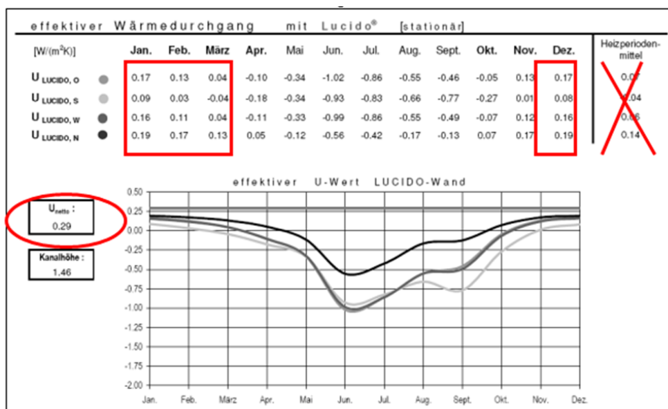
Figure 5 : Spécification de la valeur U pour les façades Lucido
