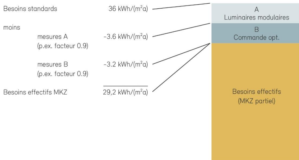
Figure 6 : Des mesures techniques d'optimisation peuvent être simplement sélectionnées, qui permettent de diminuer l'indice Minergie. Dans l'exemple, les deux mesures techniques pour la réduction de la consommation d'électricité pour l'éclairage sont appliquées à
