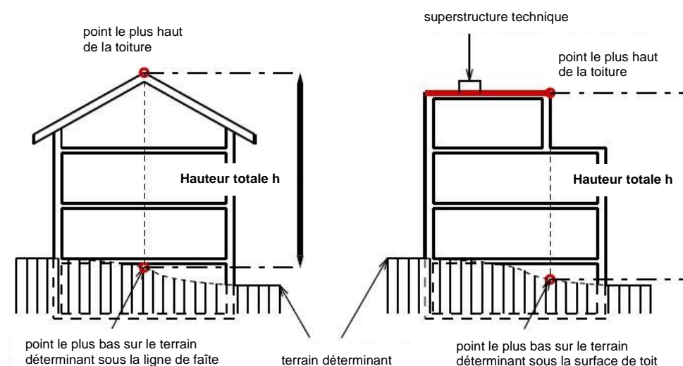
Figure 5 : définition de la hauteur totale du bâtiment
