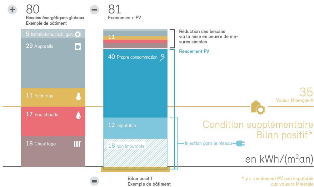
Figure 4 : Bilan et indice Minergie illustrés dans le cas d'un immeuble collectif respectant Minergie-A.
