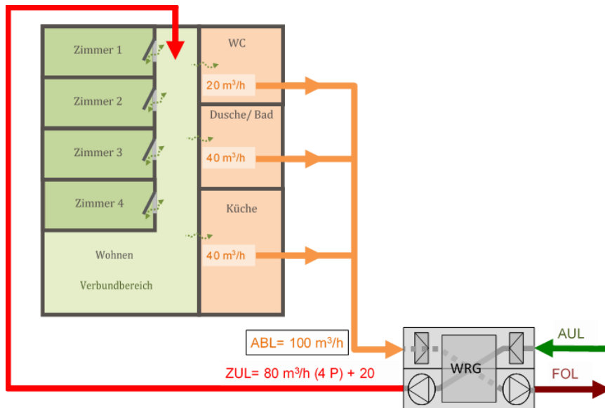
Figure 35 : exemple de ventilation de base pour les rénovations
