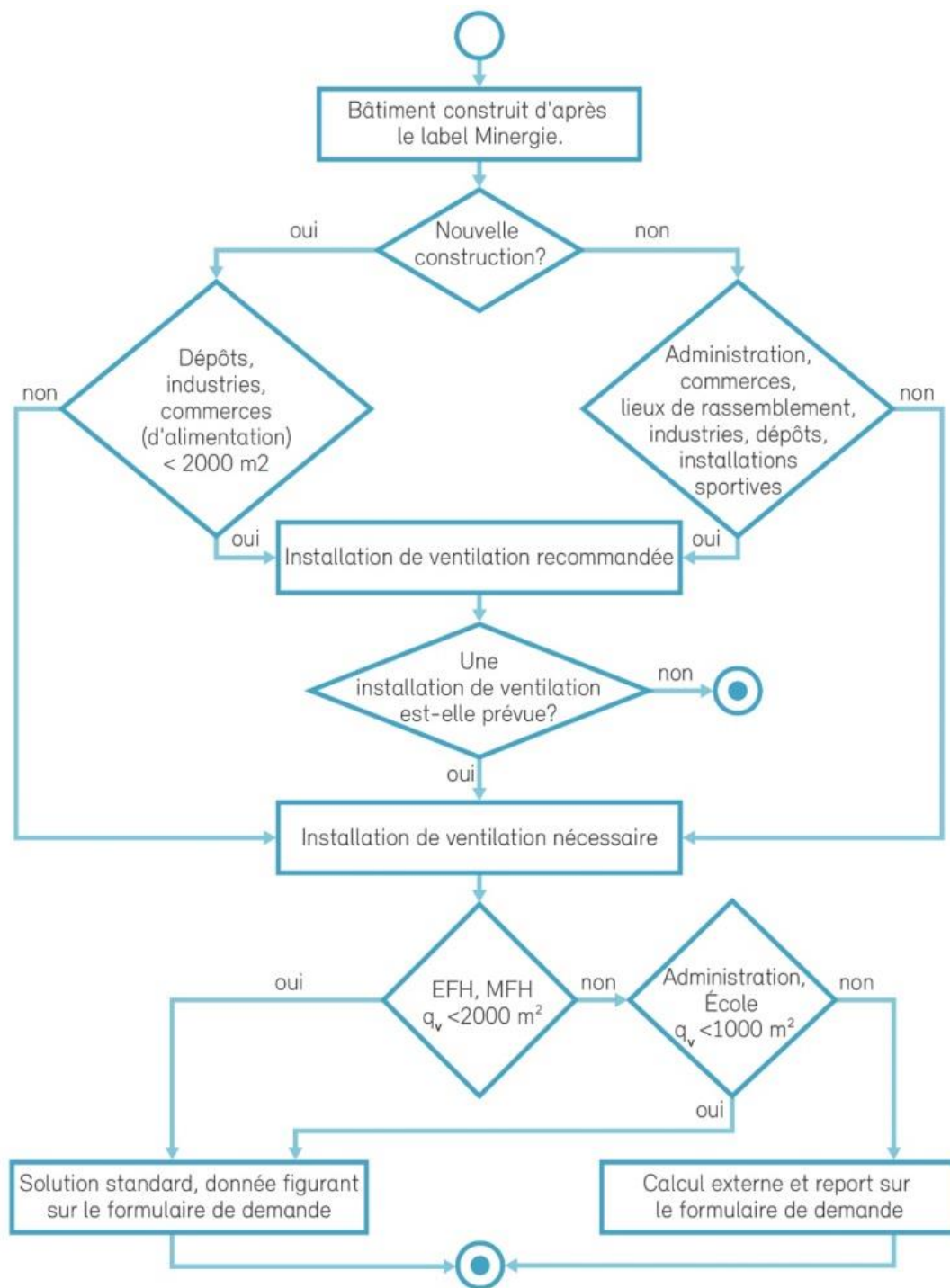
Figure 31: schéma pour évaluer si on peut se passer ou non d'une installation de ventilation
