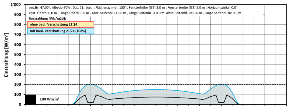
Figure 21 : diagramme d'irradiation nord le 21 juin
