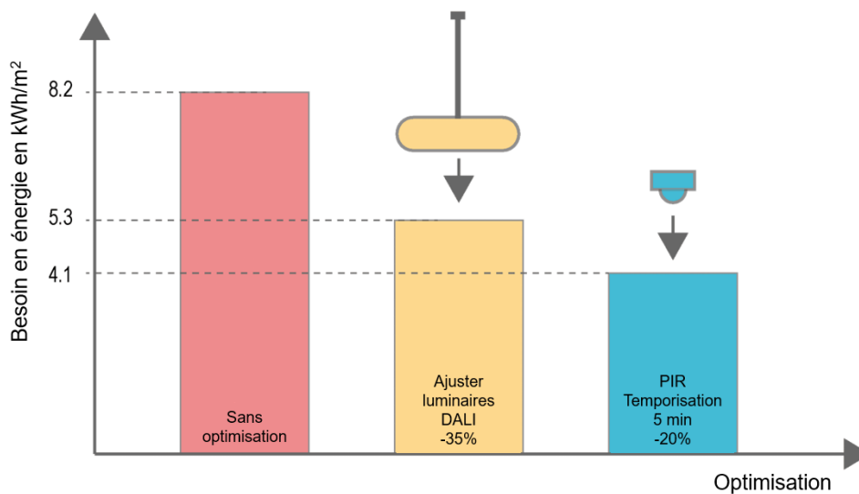
Figure 38 : Exemple "Optimisation de l'éclairage dans une école"
