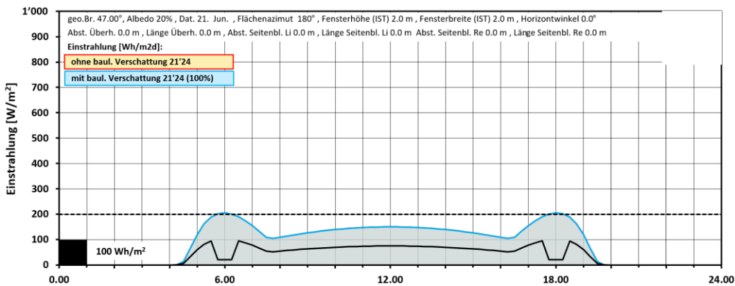
Abbildung 28: Einstrahlungsdiagramm Nord 21. Juni
