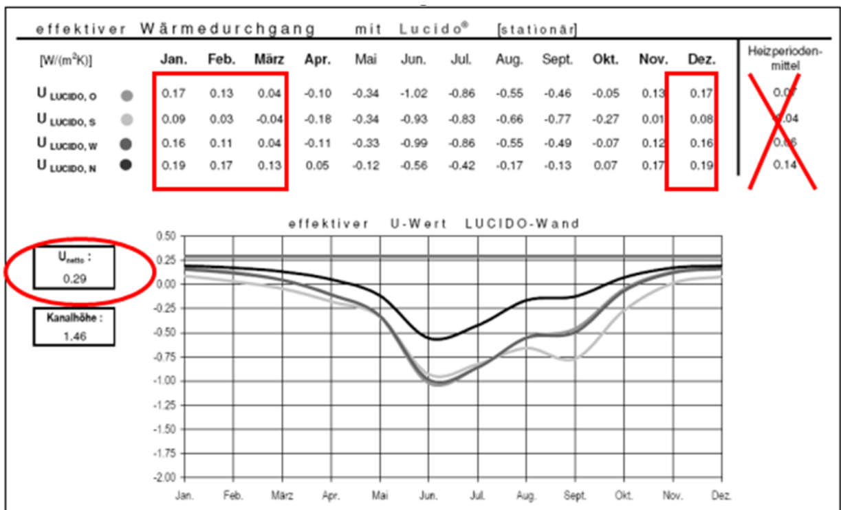
Abbildung 10: Festlegung U-Wert bei Lucido Fassade
