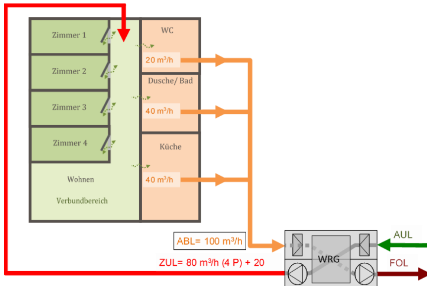
Abbildung 43: Beispiel Grundlüftung für Sanierungen
