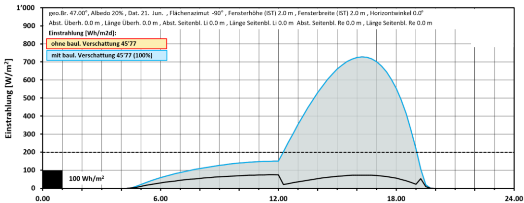
Abbildung 27: Einstrahlungsdiagramm West 21. Juni
