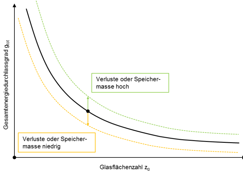
Abbildung 17: Auswirkung auf den Gesamtenergiedurchlassgrad in der raumweisen Systembetrachtung (beispielhaft)
