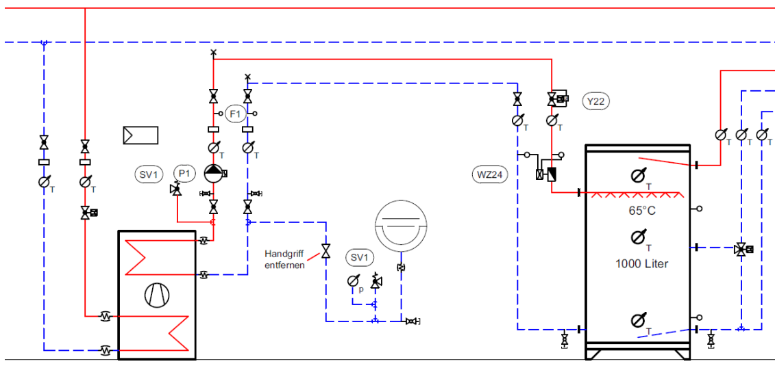
Abbildung 38: Schema Warmwasser-Booster
