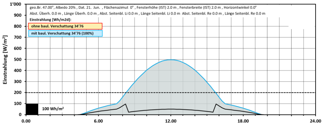
Abbildung 26: Einstrahlungsdiagramm Süd 21. Juni
