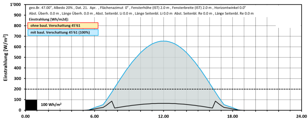
Abbildung 29: Einstrahlungsdiagramm Süd 21. April
