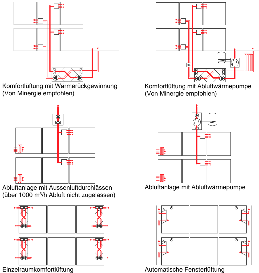
Abbildung 40: Auswahl Lüftungsanlagen für «Standard-Lüftungsanlagentyp»
