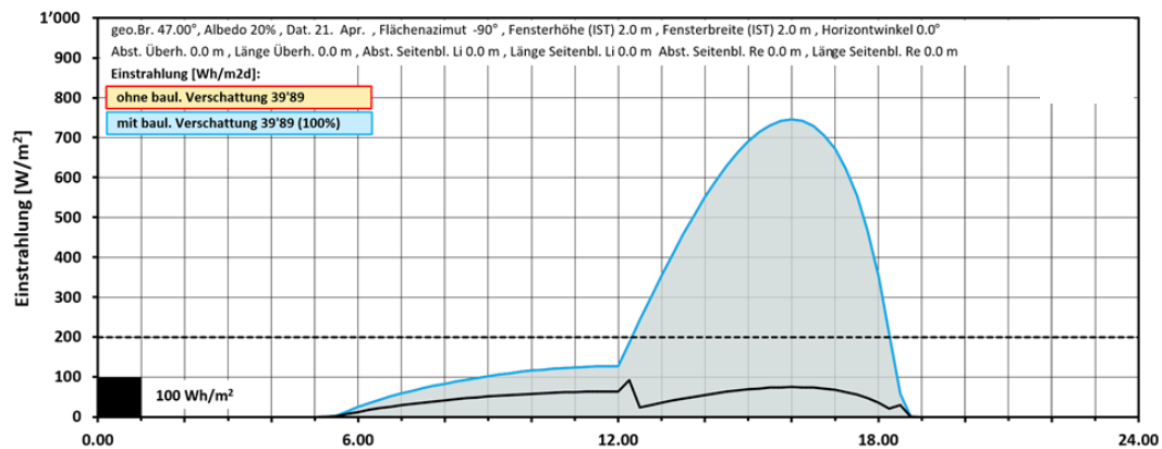
Abbildung 30: Einstrahlungsdiagramm West 21. April
