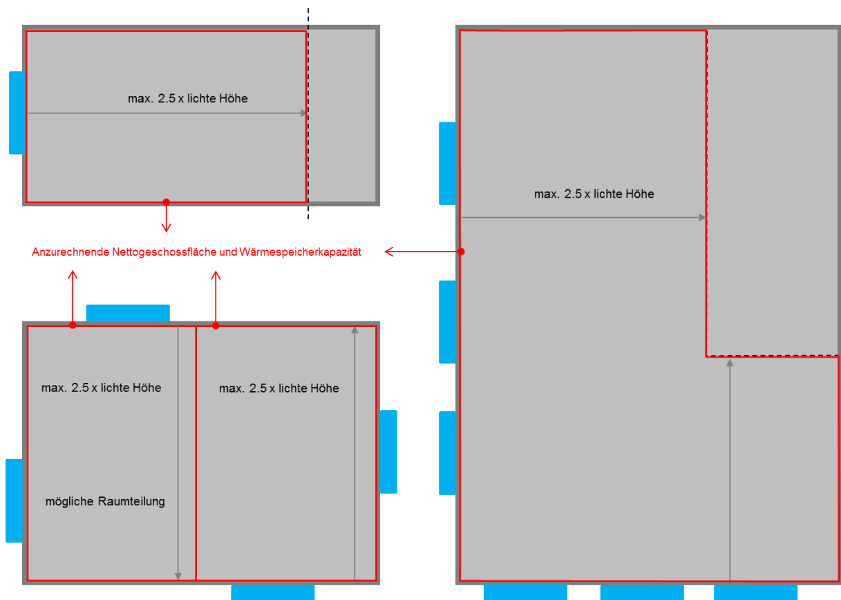
Abbildung 25: maximale anzurechnende Raumtiefe und Aufteilung von Räumen
