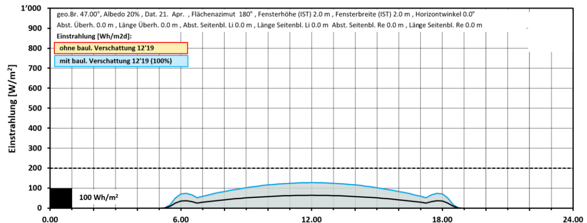
Abbildung 31: Einstrahlungsdiagramm Nord 21. April
