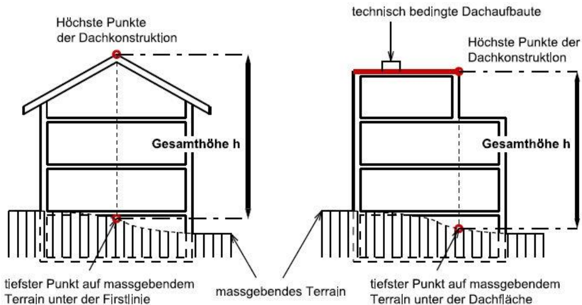
Abbildung 4: Definition Gesamthöhe Gebäude
