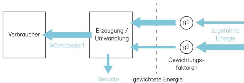
Abbildung 37: Prinzip der Energieberechnung im Minergie-Standard
