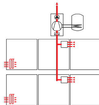
Installation d'extraction d'air avec pompe à chaleur
