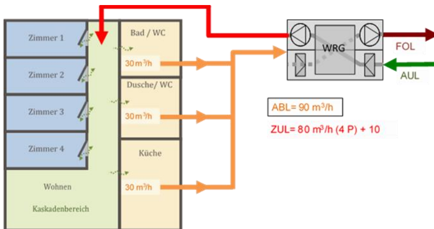
Figure 34: Exemple de ventilation de base pour des rénovations
