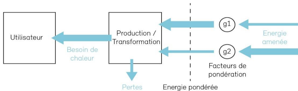
Figure 28 : Schéma de principe du réseau d'anergie
