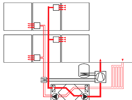
Aération douce avec pompe à chaleur sur air sortant (recommandé par Minergie)
