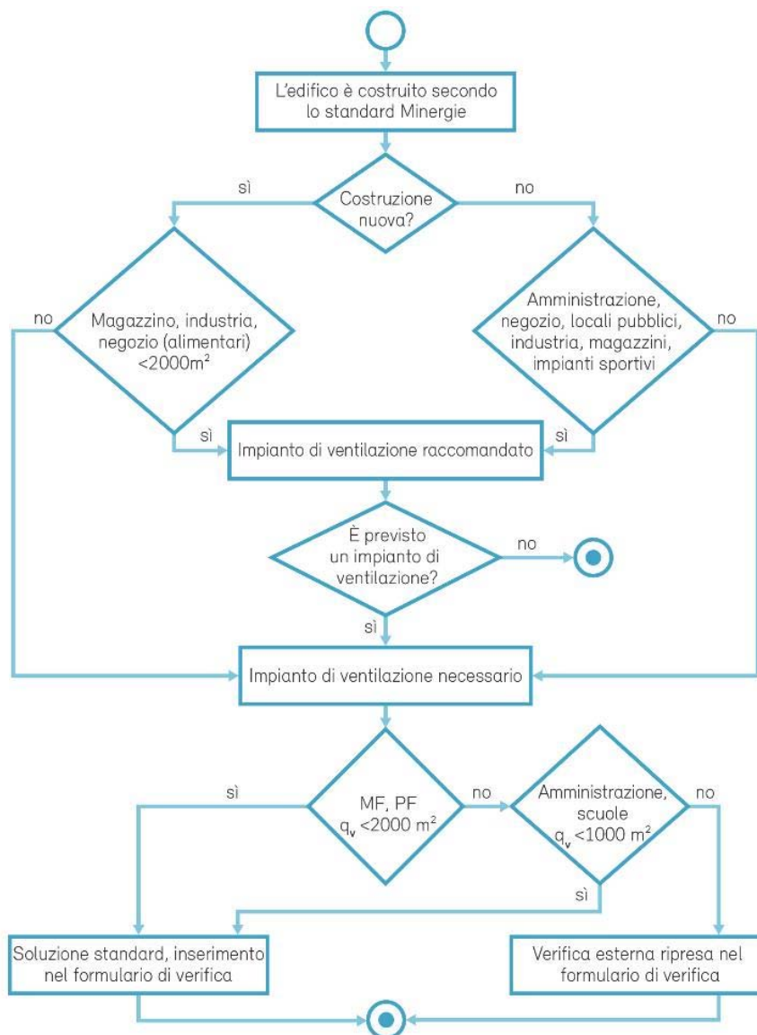
Figura 31: Diagramma di flusso per determinare se è possibile rinunciare a un sistema di ventilazione controllata
