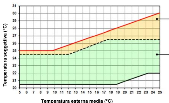
Figura 20: Confronto delle esigenze secondo la SIA 180
