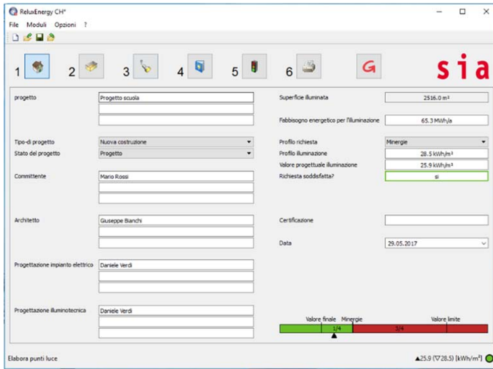
Figura 38: foglio del risultato di ReluxEnergy
