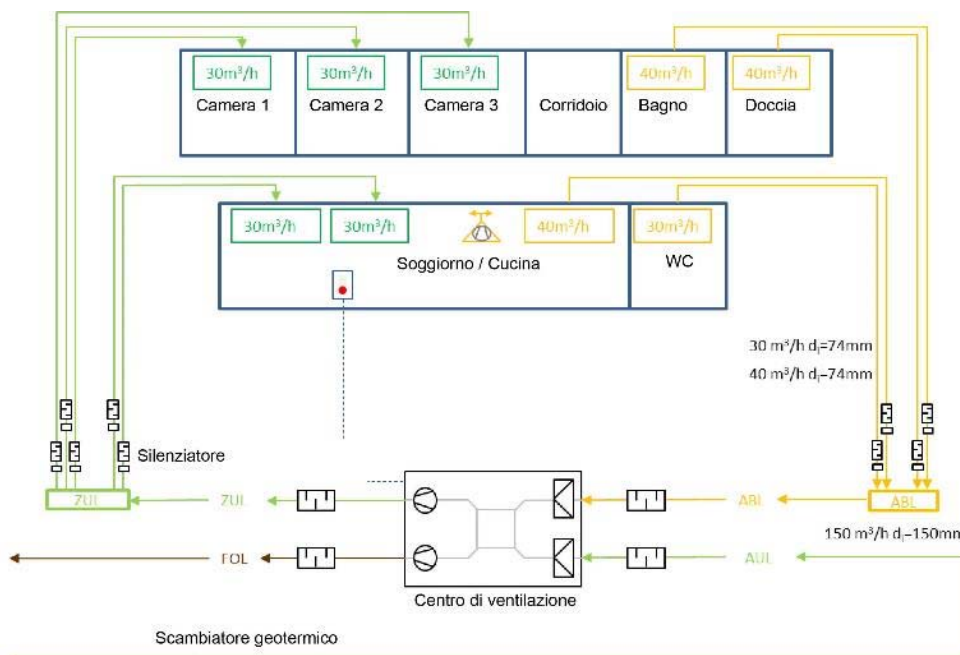
Figura 34: Esempio schema di ventilazione per piccoli impianti
