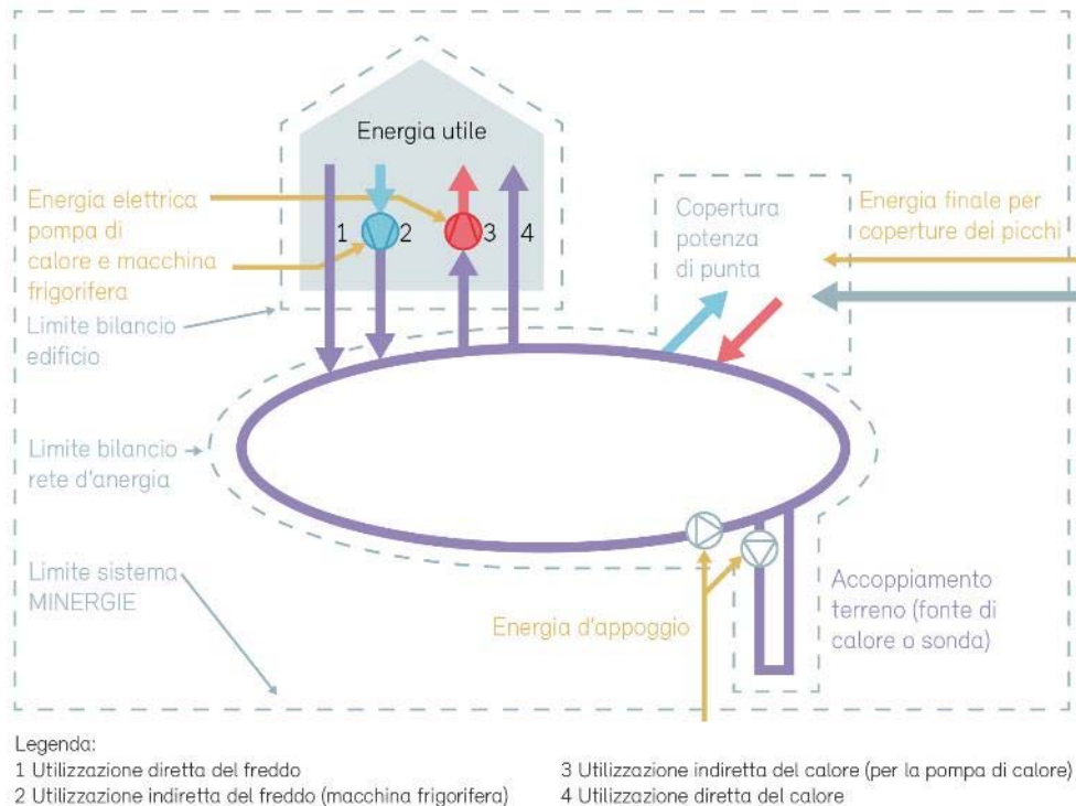
Figura 28: schema di principio di una rete d'energia
