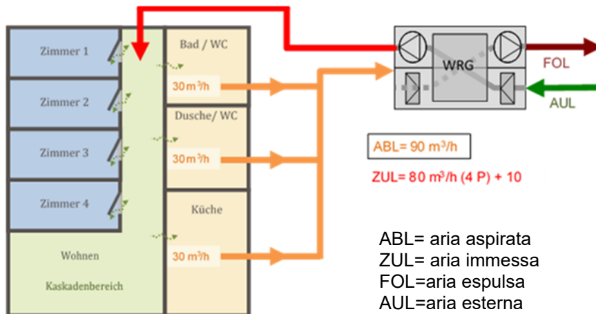
Figura 35: esempio di ventilazione controllata per risanamenti
