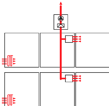
Estrazione dell'aria con bocchette d'immissione d'aria esterna
