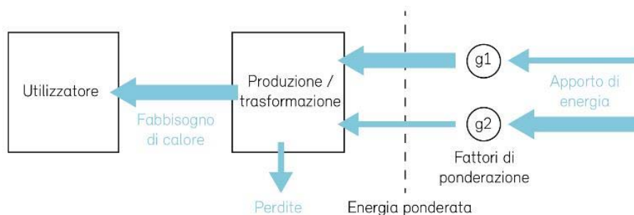
Figura 29: Principio di calcolo dell'energia nello standard Minergie
