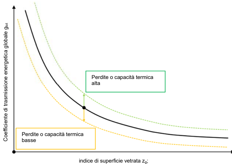
Figura 14: Effetto sul coefficiente di trasmissione energetica globale nella verifica di sistema individuale per locale (esempio)
