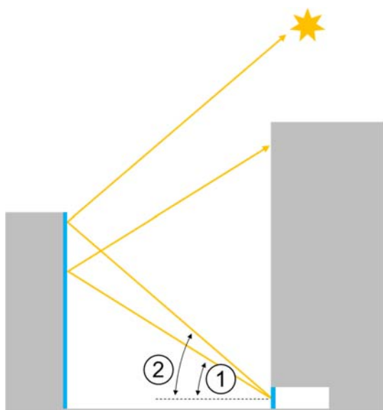
Figura 18: Possibili angoli d'irraggiamento rispettivamente rapporti visivi
