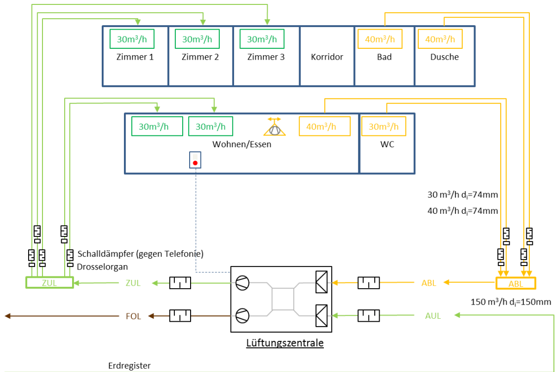
Abbildung 34: Beispiel Lüftungsschema für Kleinanlagen
