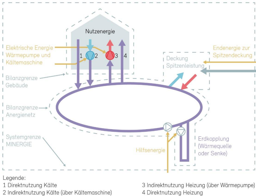
Abbildung 28: Prinzipskizze Anergienetz
