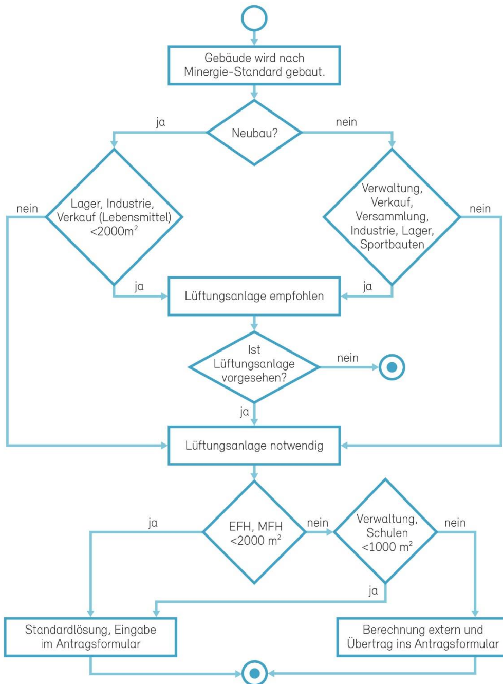
Abbildung 31: Ablaufdiagramm zur Eruiierung ob auf eine Lüftungsanlage verzichtet werden kann
