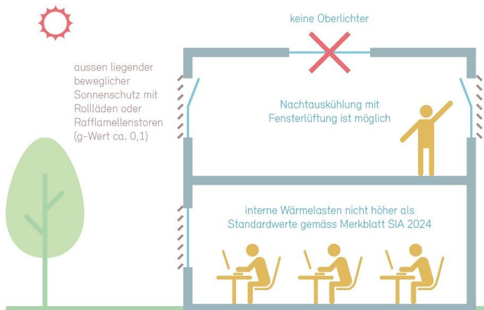
Abbildung 11: Rahmenbedingungen für Variante 1
