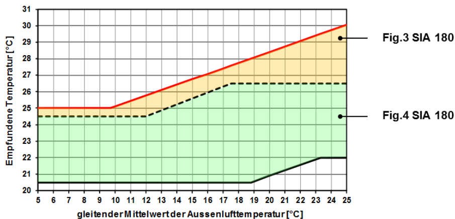
Abbildung 21: Fig. 3 und Fig.4 nach SIA 180
