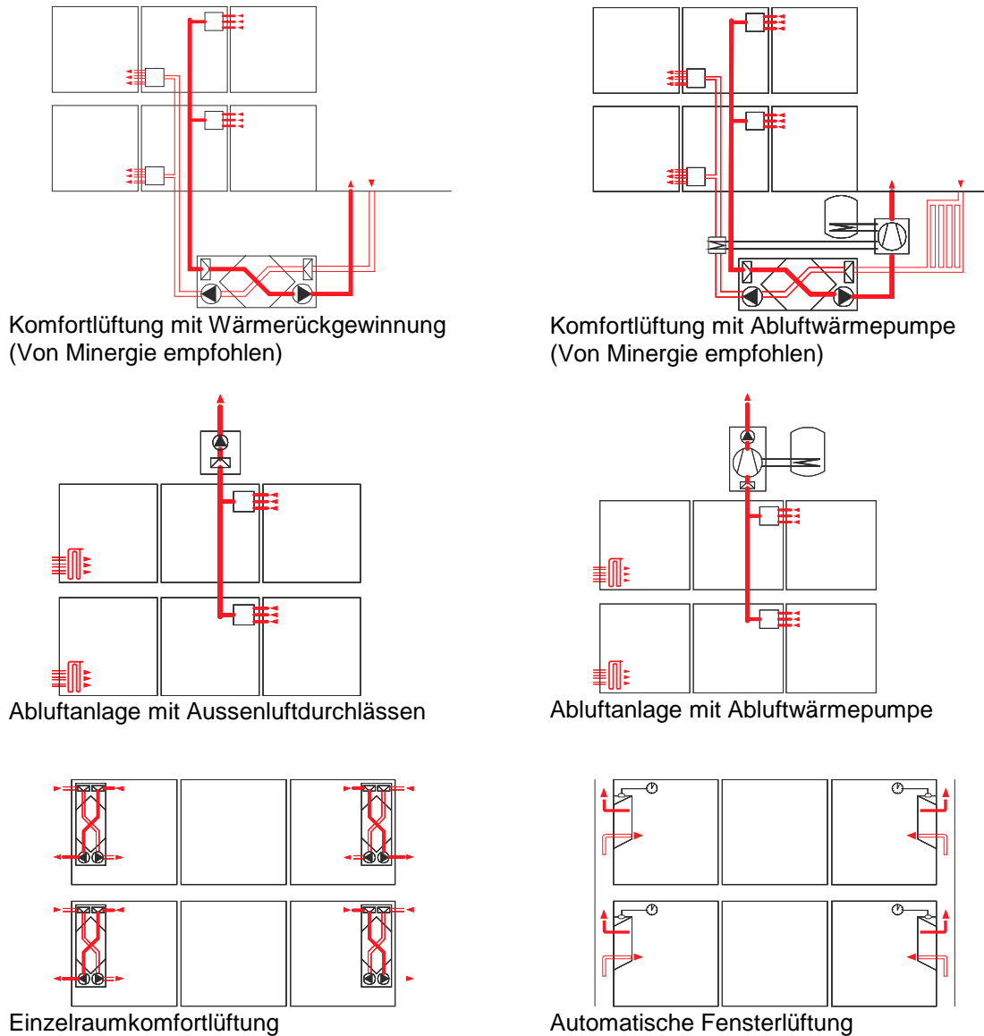
Abbildung 32: Auswahl Lüftungsanlagen für «Standard-Lüftungsanlagentyp»
