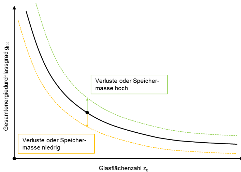
Abbildung 14: Auswirkung auf den Gesamtenergiedurchlassgrad in der raumweisen Systembetrachtung (beispielhaft)
