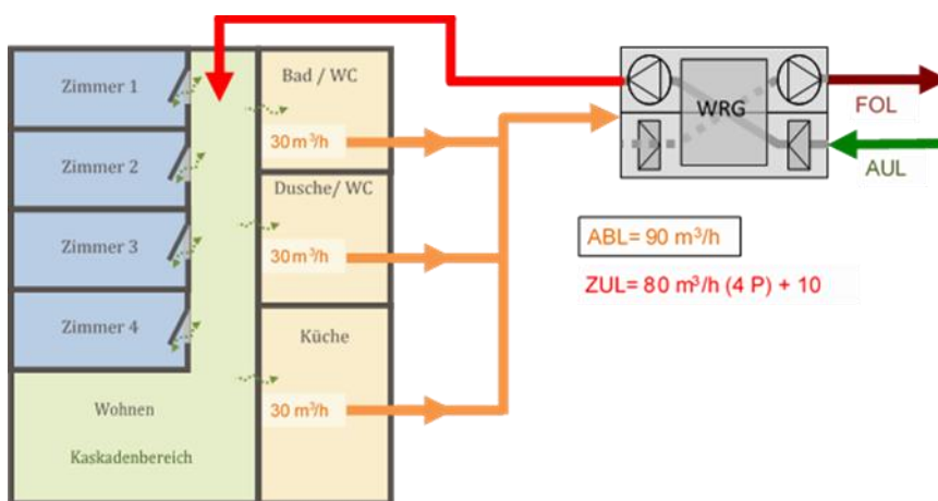
Abbildung 35: Beispiel Grundlüftung für Sanierungen
