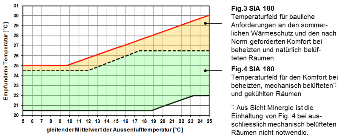
Abbildung 10: Vergleich Anforderungen nach SIA 180
