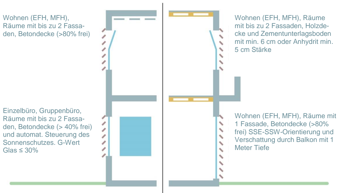
Abbildung 12: Standardfälle für Wohnbauten (Variante 1)
