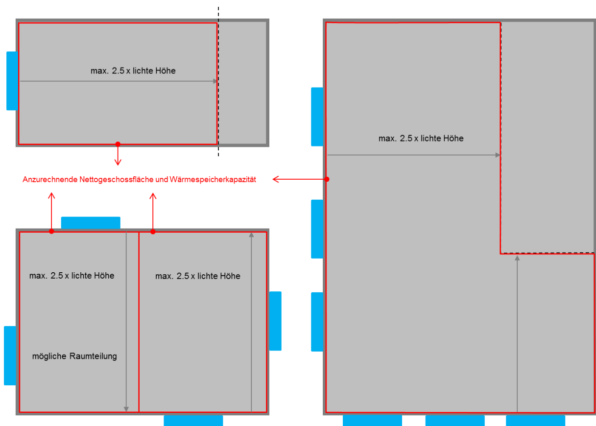
Abbildung 22: maximale anzurechnende Raumtiefe und Aufteilung von Räumen
