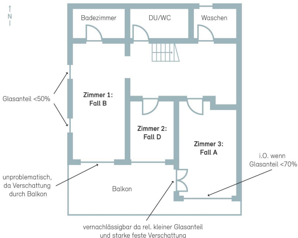
Abbildung 23: Beispiel Einfamilienhaus Obergeschoss.
