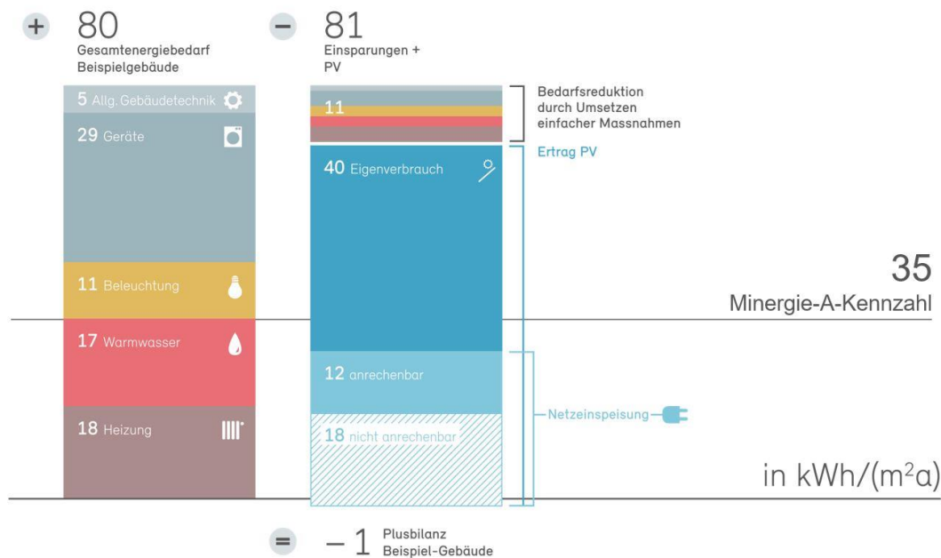
Abbildung 3: Bilanz und Minergie-Kennzahl am Beispiel eines Mehrfamilienhauses im Minergie-A-Standard
